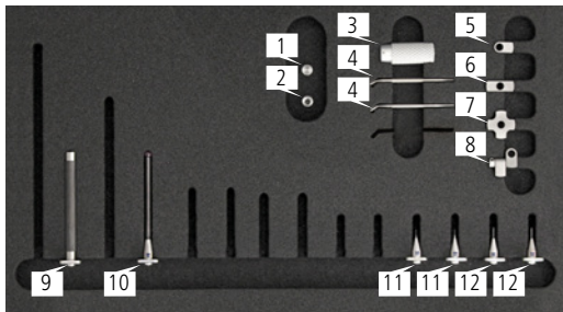
VAST XXT Tasterbausatz 4, klein, 15-teilig 626103-9024-000
